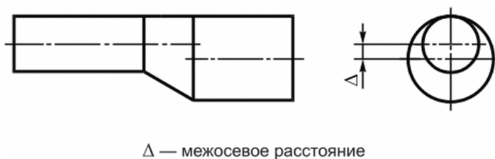
Рисунок 6.1 - Устройство несоосного перехода труб
